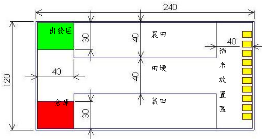
圖一 競賽場地平面圖
